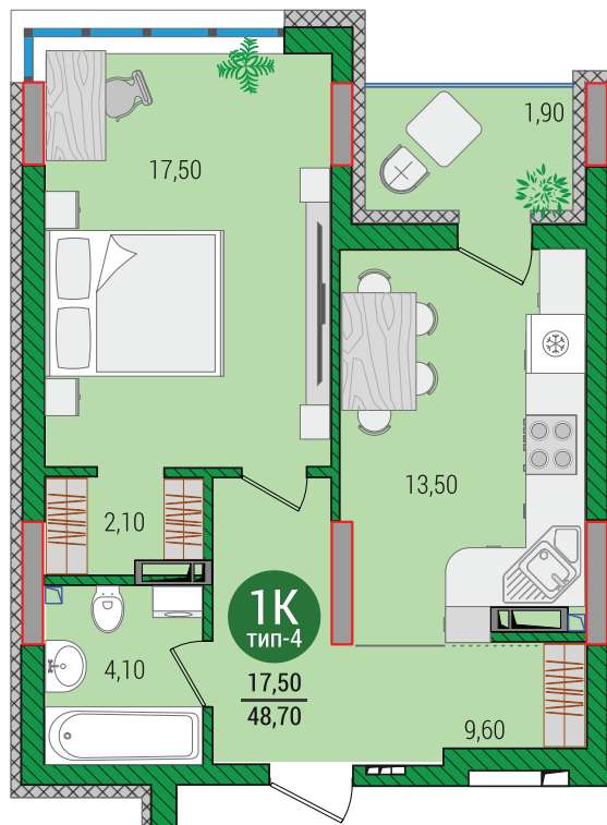
Схема розташування квартири в будинку
